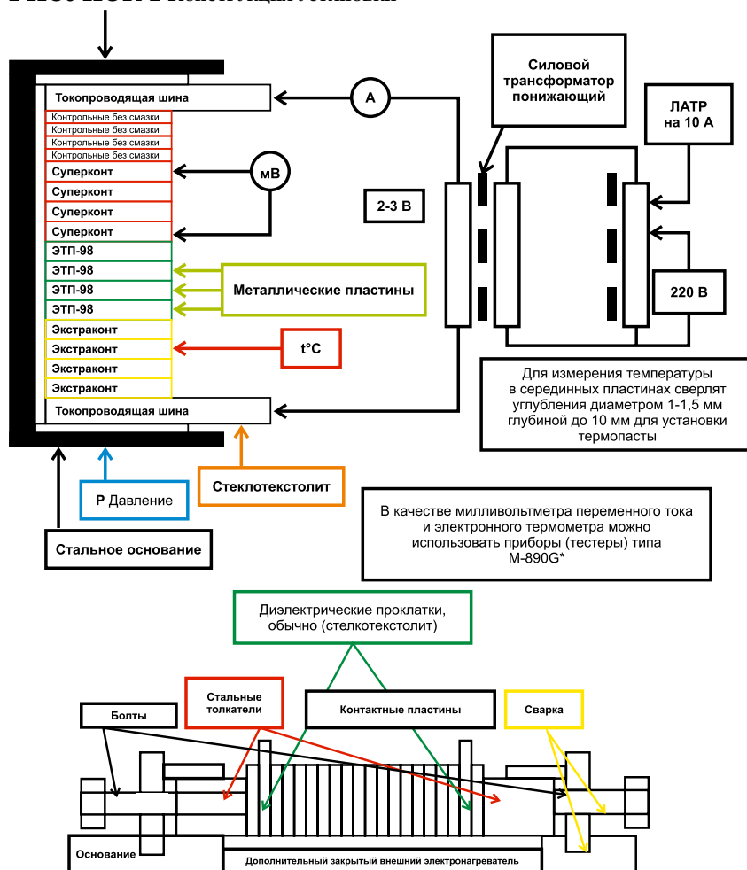
РИСУНОК 1 Конструкция установки
